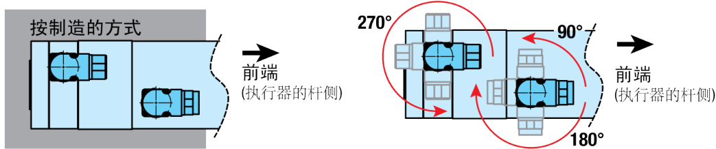
图 5.2: 连接器的旋转。请注意，Tolomatic 标准连接器可以从-90° 到+180° 旋转，允许电缆朝前（如制造的杆端），连接到电动缸的任何一侧，两侧，或背面。
