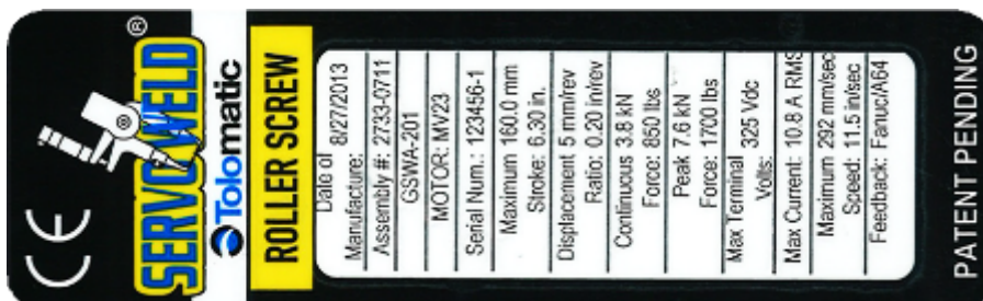
图 2.2: ServoWeld GSWA 电动缸的识别标签。
