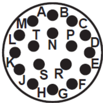
电机电源连接器
